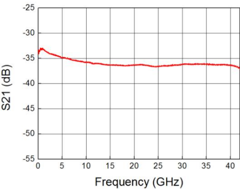
PD40G-M 频率响应曲线
