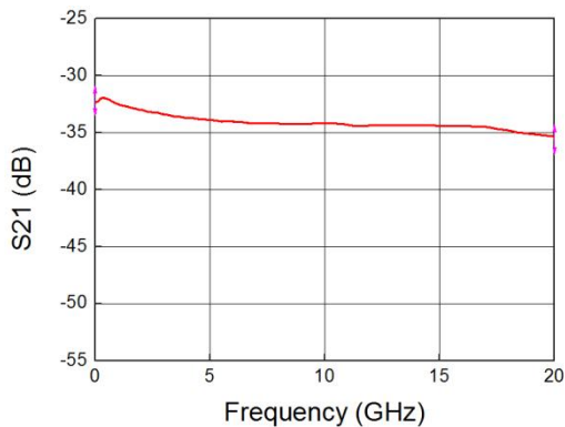
PD18G-M 频率响应曲线
