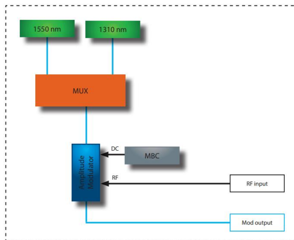
功能结构图
