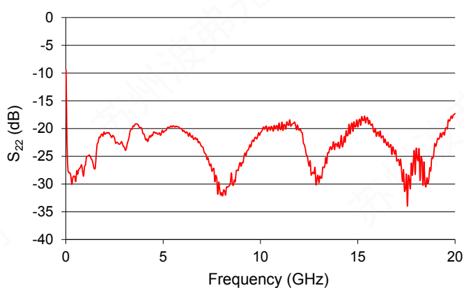
S_{22} Parameter Curve
